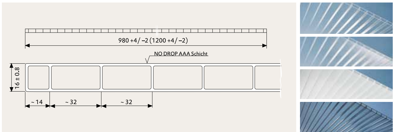
Querschnitt der PLEXIGLAS RESIST® AAA SDP 16 (Maße in mm)
