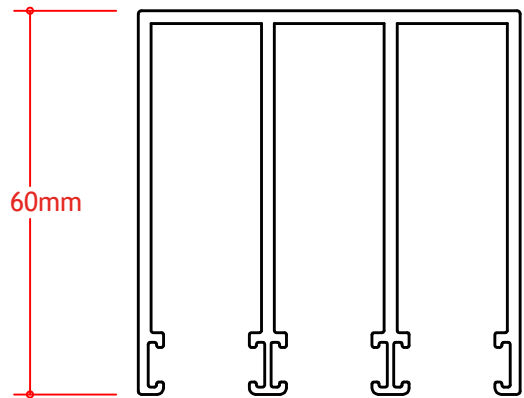
Oberprofil
