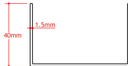
U-Profil
