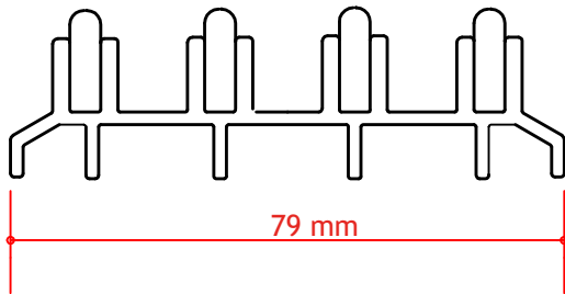
Unterprofil
